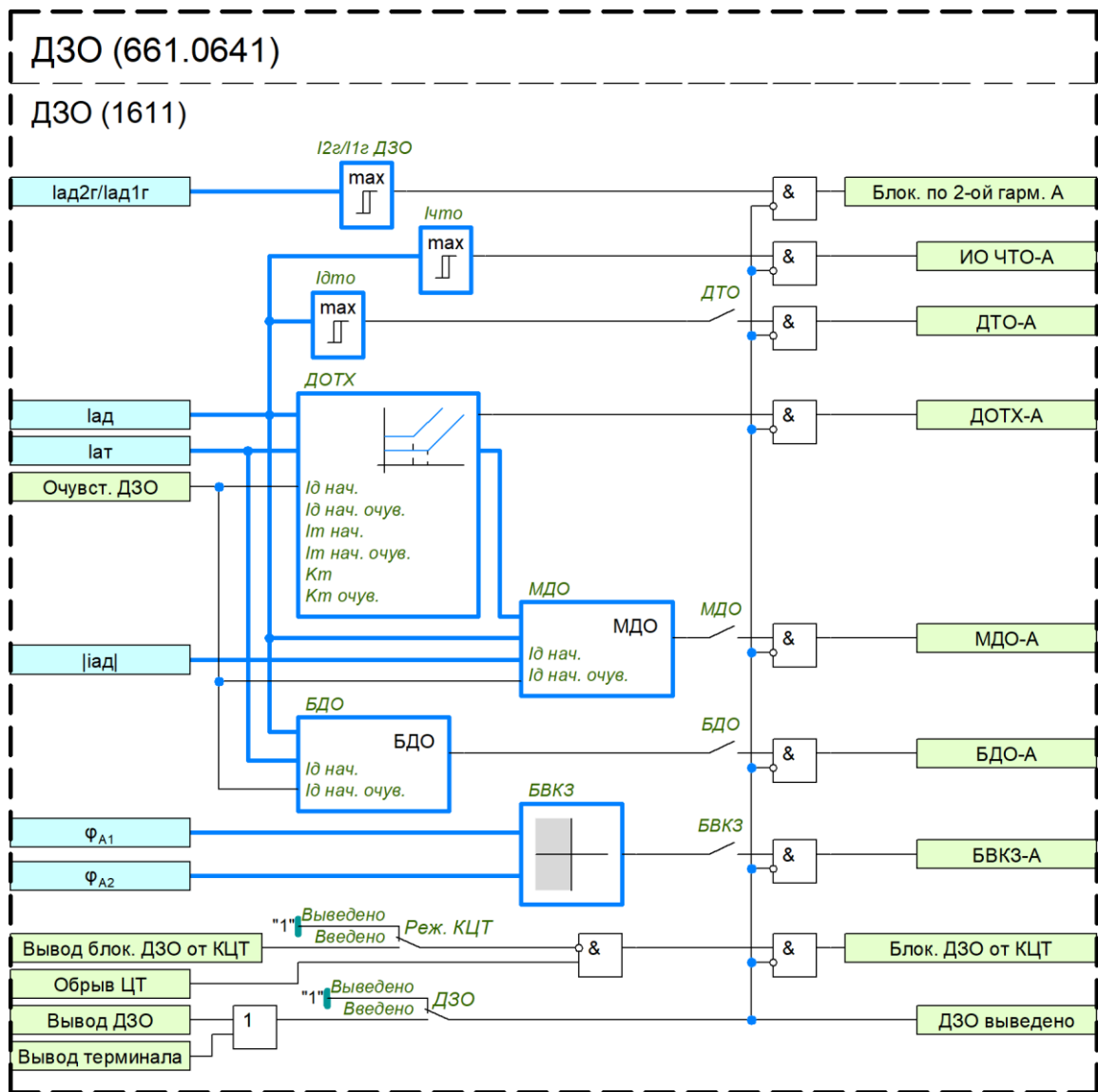
Рисунок 1 – Функциональный блок ИО ДЗО для фазы А
