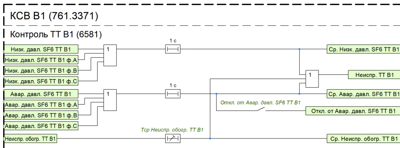
Рисунок 18 – Функциональный блок контроля исправности ТТ В1
