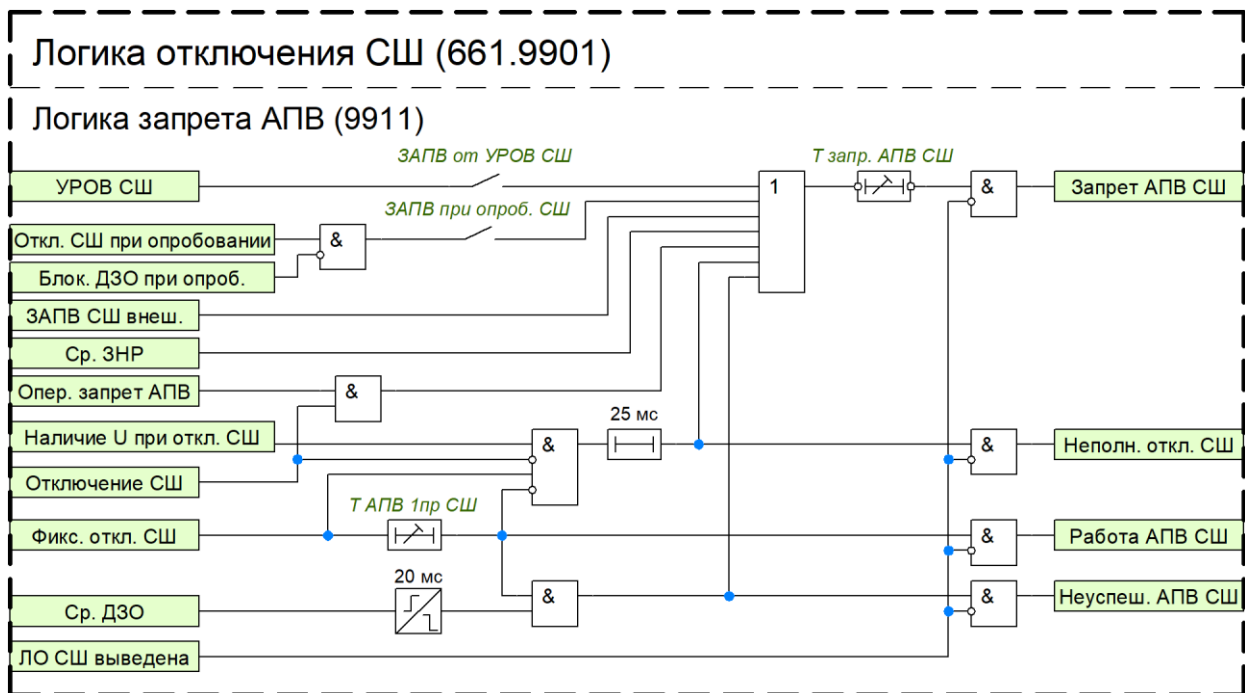
Рисунок 24 – Функциональный блок логики запрета АПВ
