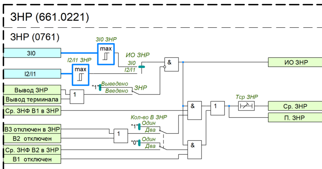
Рисунок 12 – Функциональный блок ЗНР
