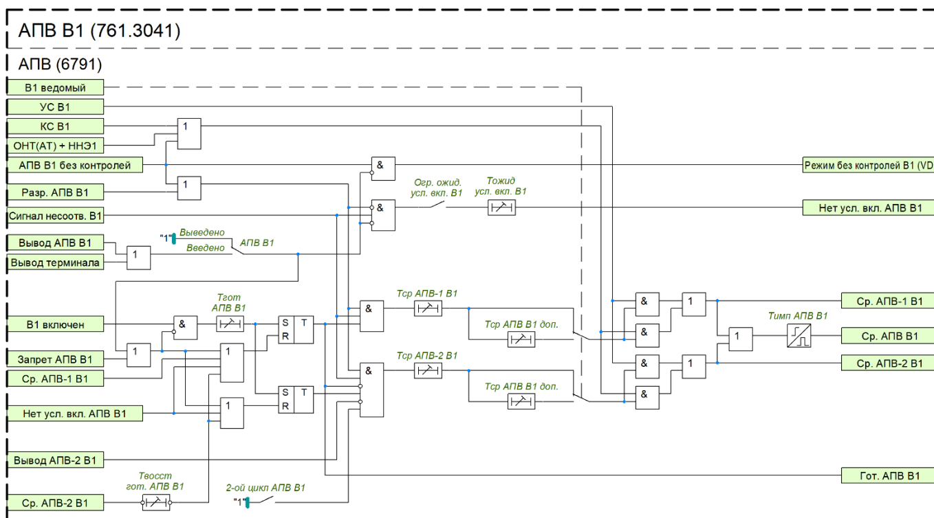
Рисунок 15 – Функциональный блок АПВ В1
