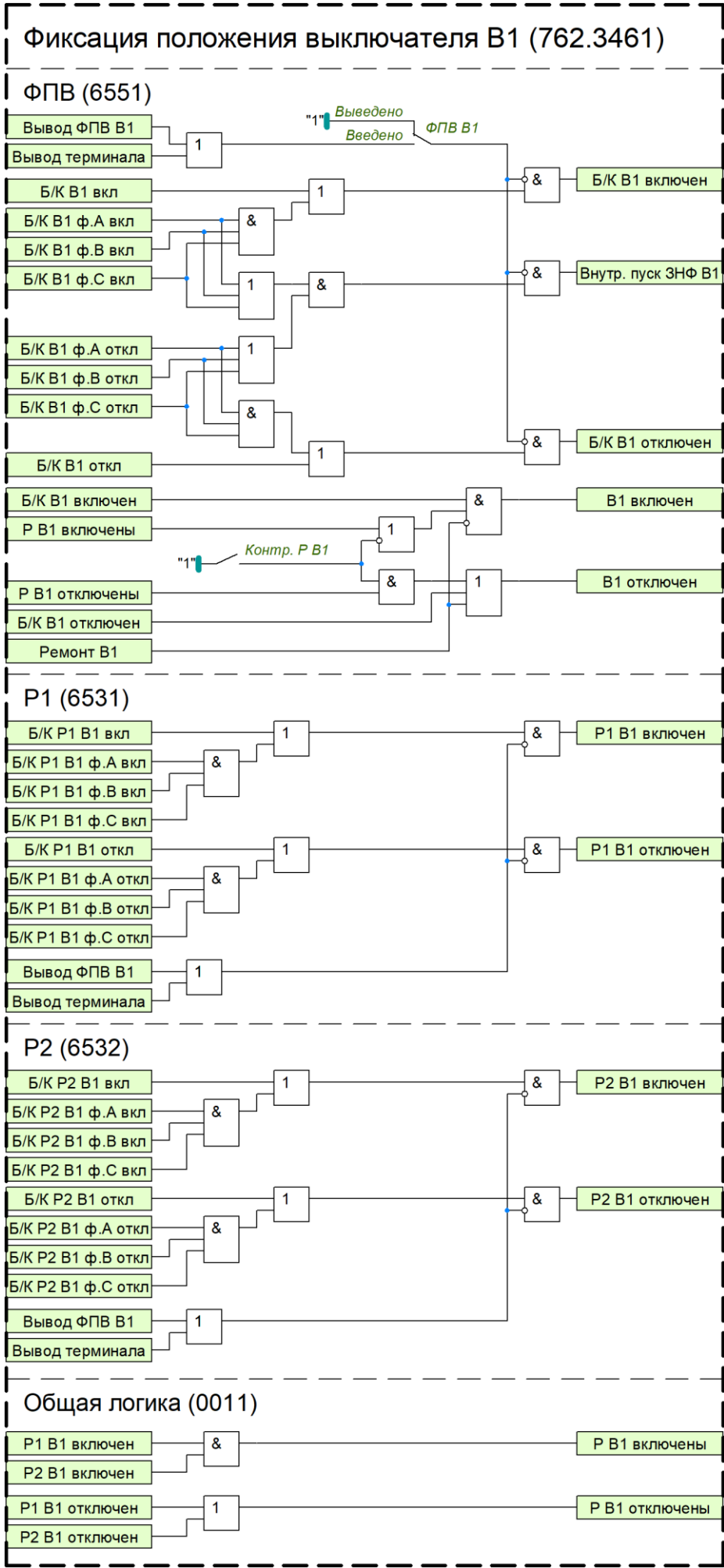
Рисунок 16 – Функциональный блок ФПВ В1
