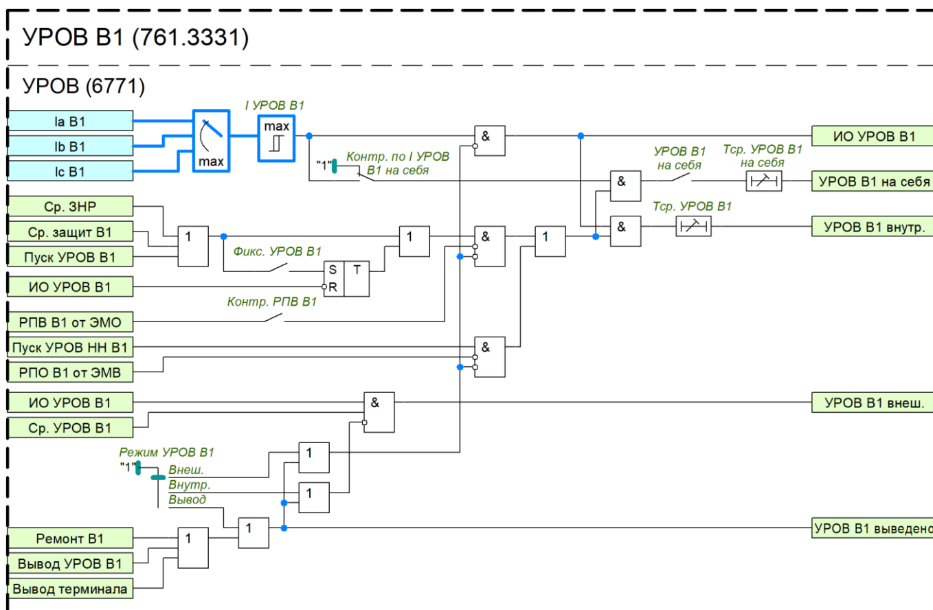
Рисунок 9 – Функциональный блок УРОВ В1
