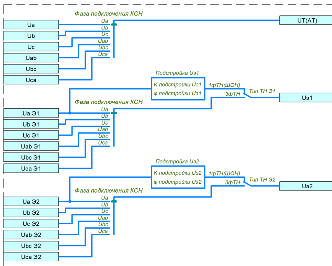
Рисунок 13 – Выбор величин напряжений для КСН
