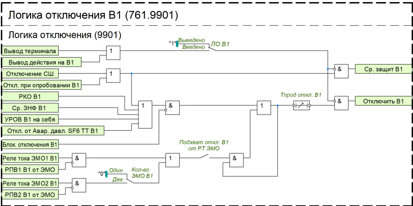
Рисунок 27 – Функциональный блок логики отключения В1
