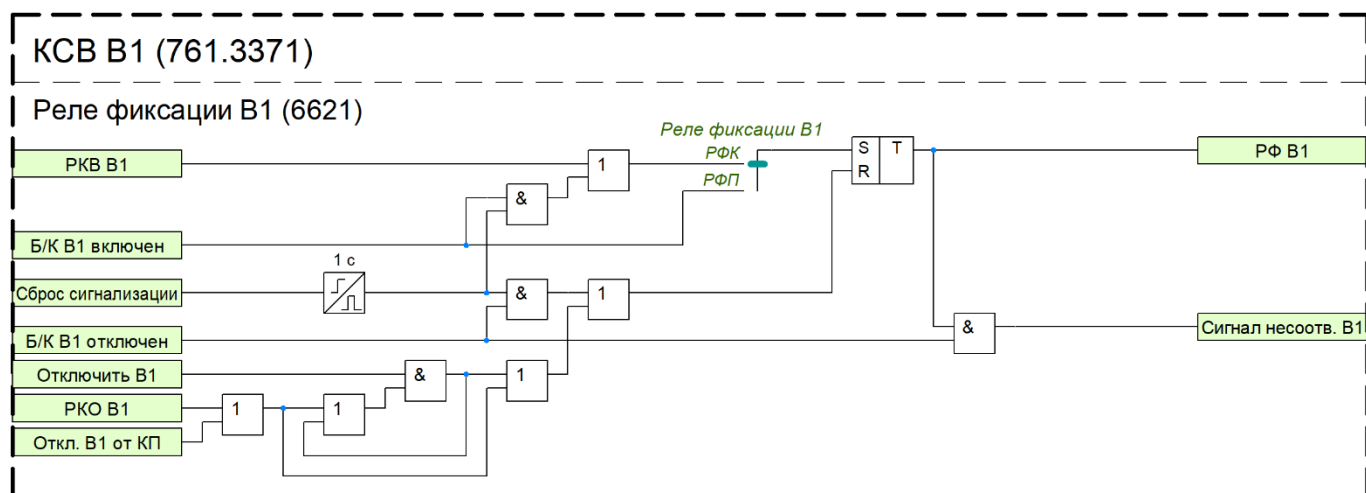
Рисунок 22 – Функциональный блок реле фиксации В1
