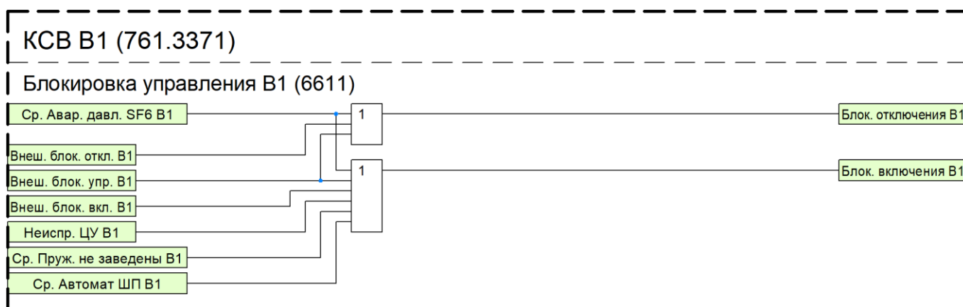
Рисунок 21 – Функциональный блок блокировки управления В1
