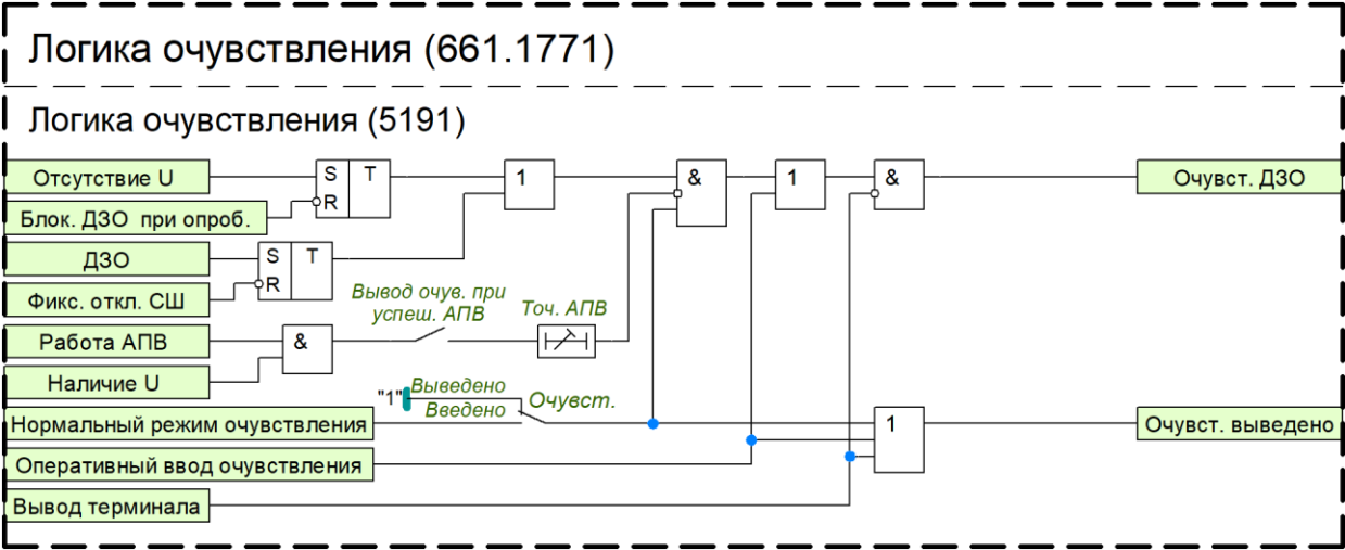
Рисунок 8 – Функциональный блок логики очувствления
