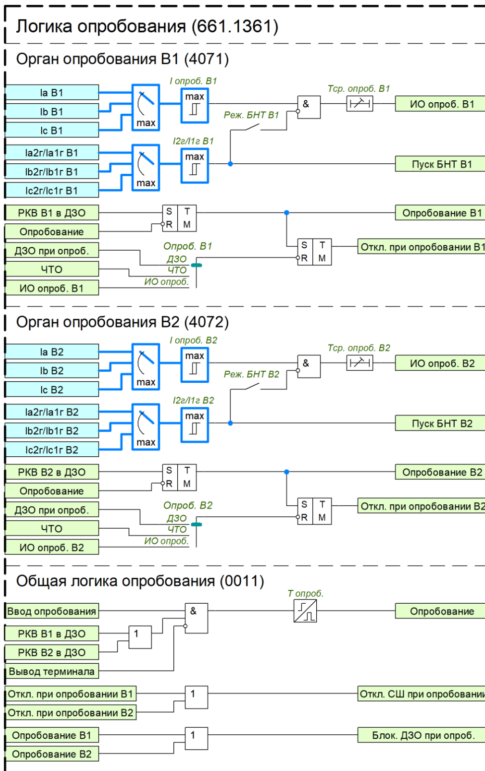
Рисунок 7 – Функциональный блок логики опробования
