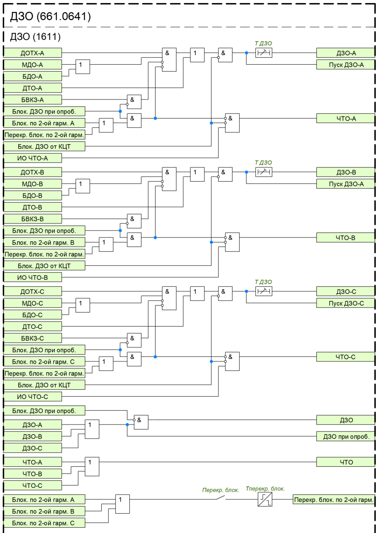
Рисунок 4 – Функциональный блок ДЗО
