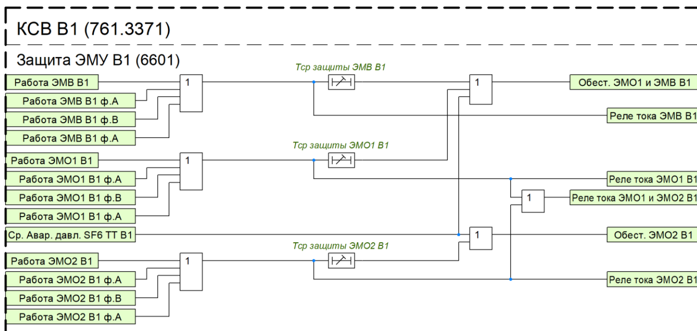
Рисунок 20 – Функциональный блок защиты ЭМУ В1 от длительного протекания тока
