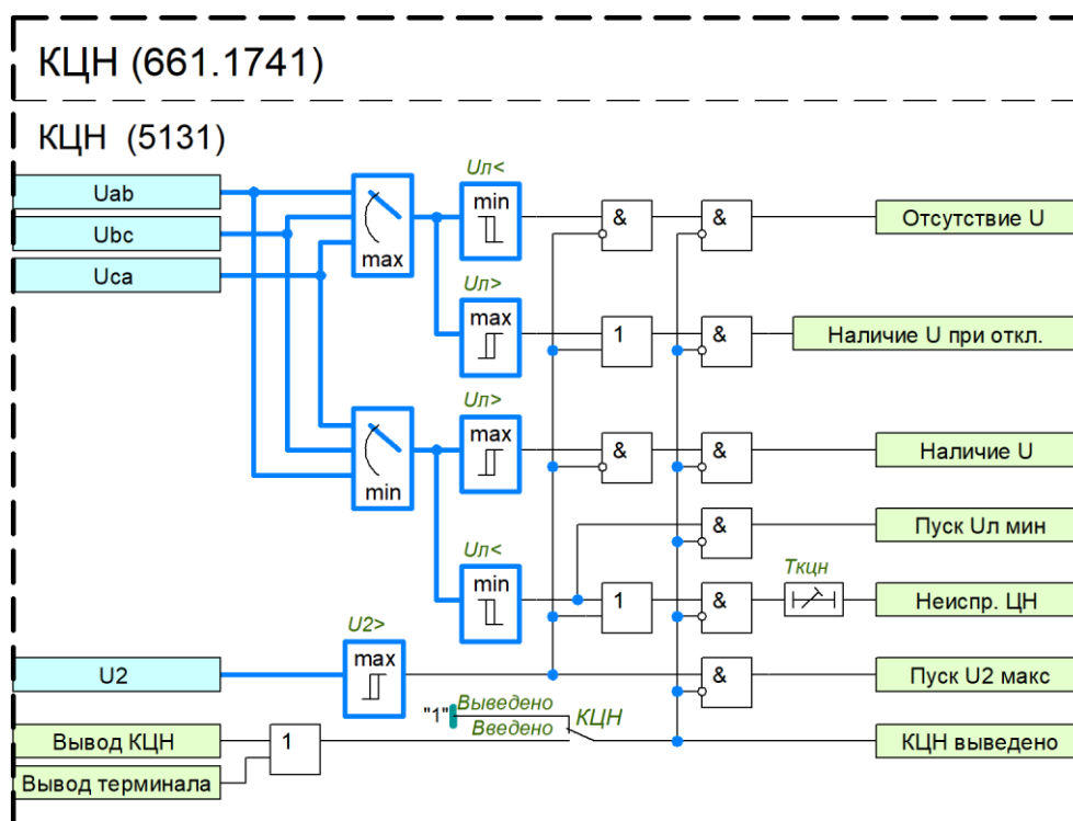
Рисунок 6 – Функциональный блок КЦН
