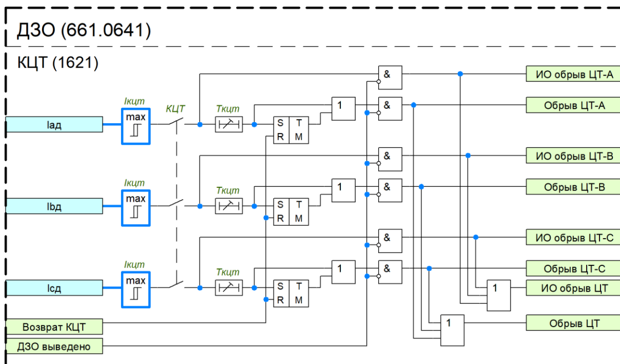
Рисунок 5 – Функциональный блок КЦТ
