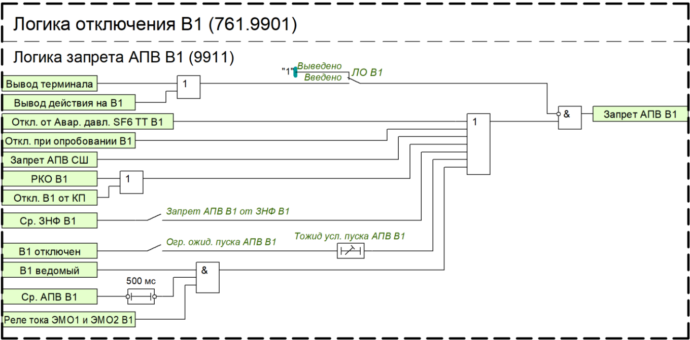
Рисунок 26 – Функциональный блок логики запрета АПВ В1
