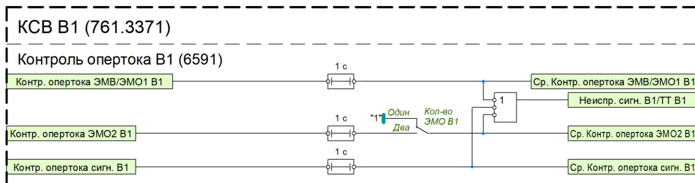
Рисунок 19 – Функциональный блок контроля оперативного тока цепей сигнализации В1
