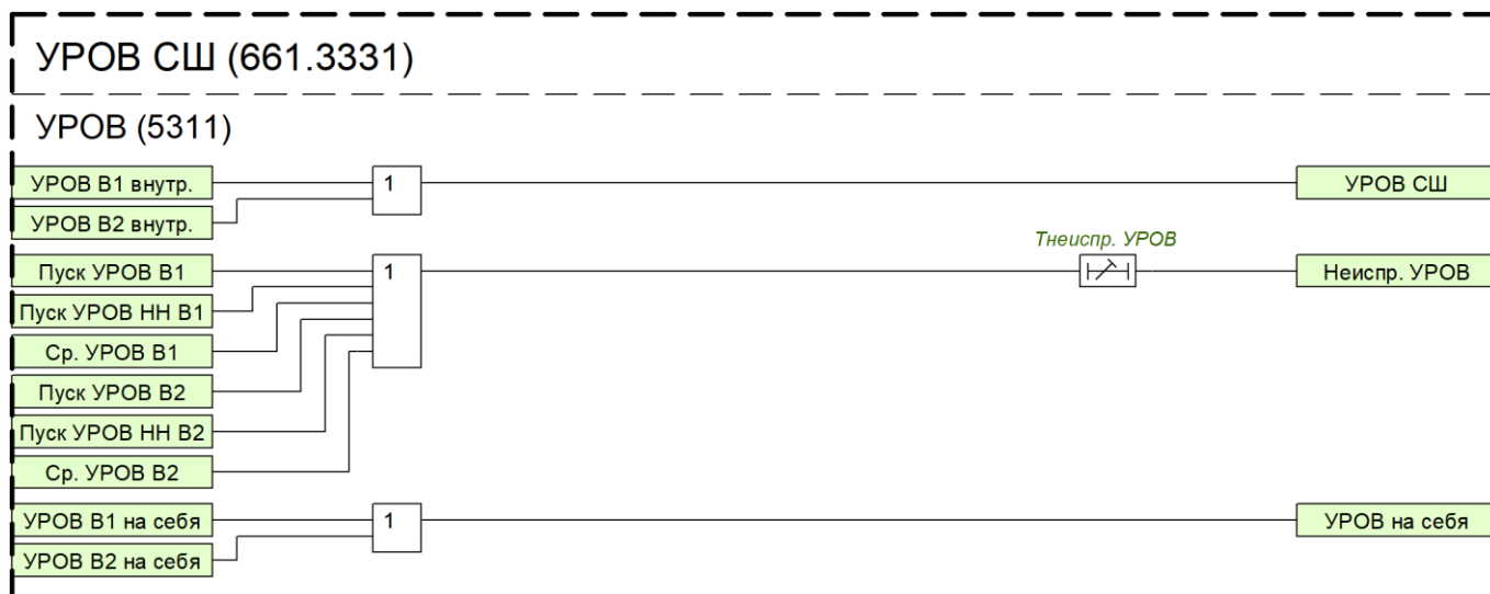
Рисунок 10 – Функциональный блок УРОВ СШ
