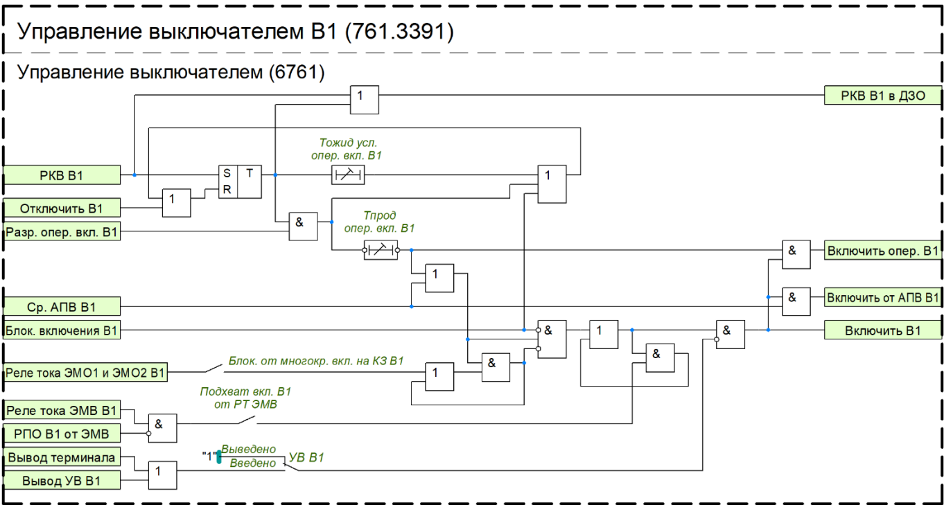
Рисунок 23 – Функциональный блок управление выключателем В1
