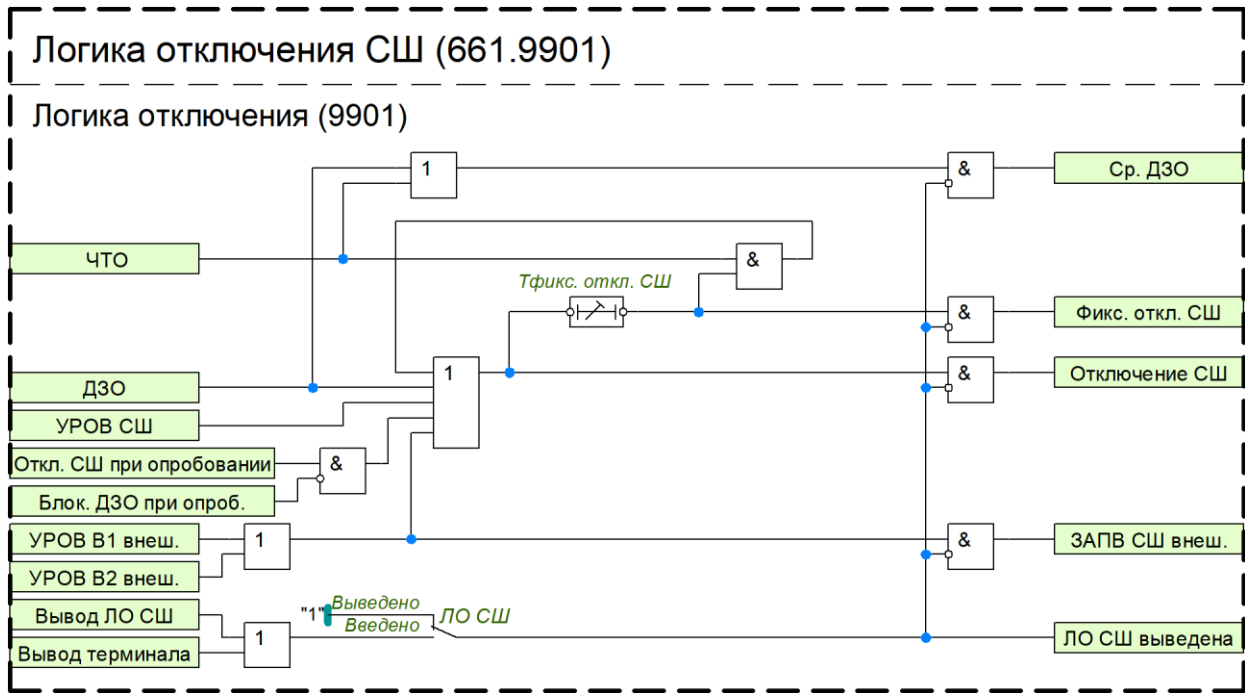
Рисунок 25 – Функциональный блок логики отключения ошиновки
