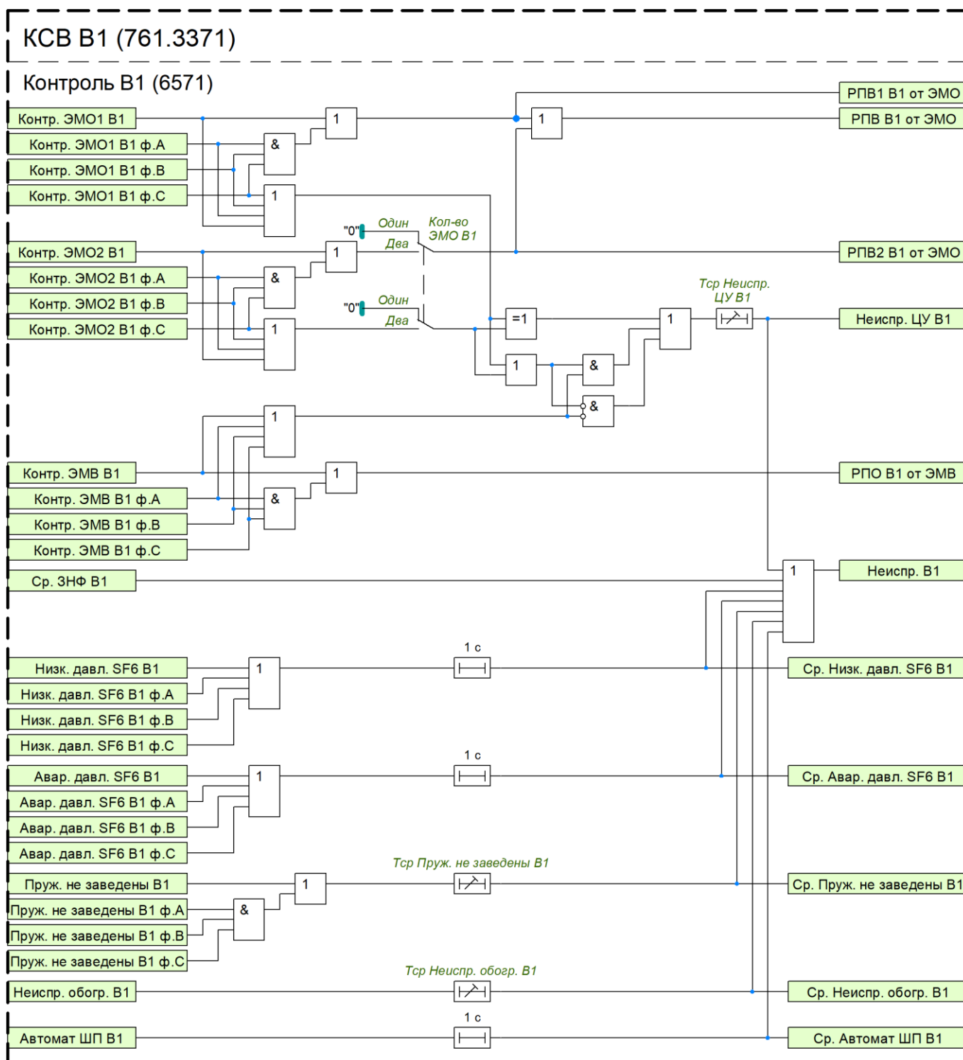
Рисунок 17 – Функциональный блок контроля исправности выключателя В1
