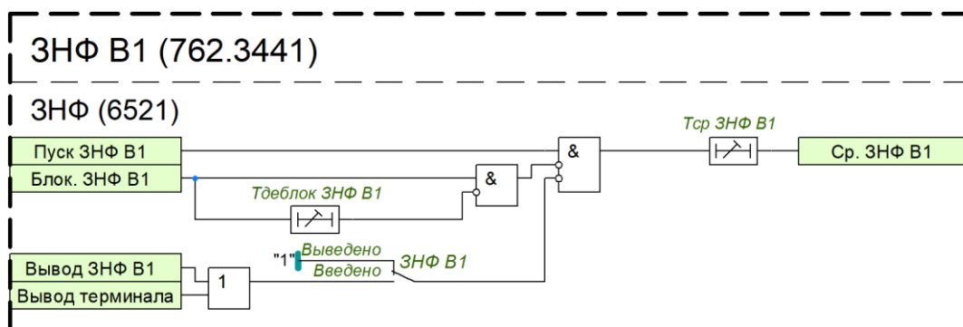
Рисунок 11 – Функциональный блок ЗНФ В1
